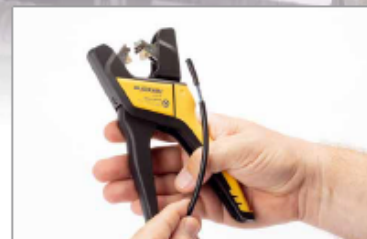
So soll es aussehen. Eine sauber geschnittene Außenisolierung und unverletzte Innelleiter
