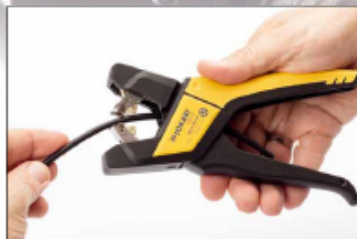
Durch die nach hinten offene Zange kann bei Bedarf auch lang abgemantelt werden
