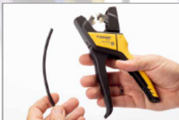
Die Sensor Special nimmt Kabeldurchmesser von 4,4 bis 7 mm auf
